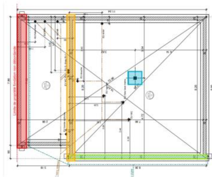
Figure 1 : Plan de fondation – éléments de soubassement.
